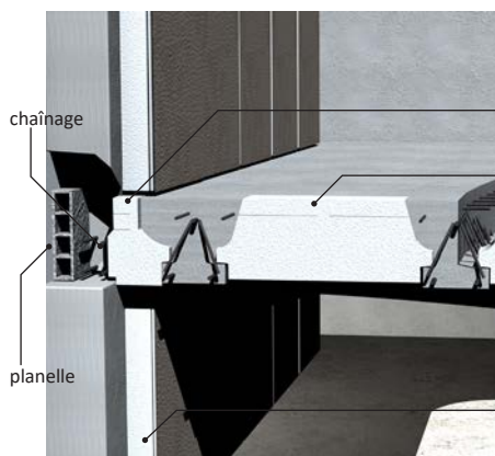
cas n°1 rupteur total (prévoir un écran feu sous les rupteurs)
